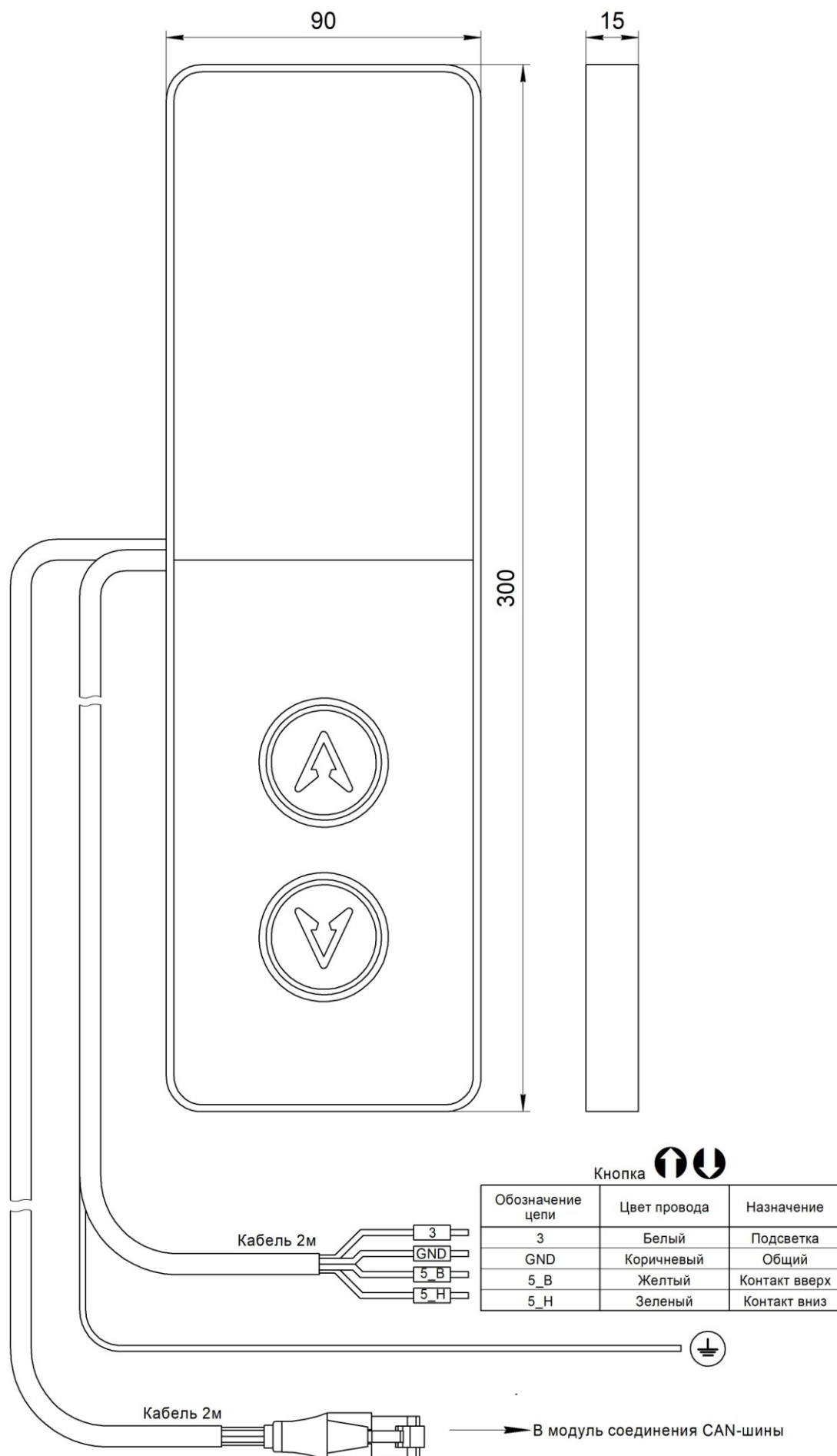
Рис.1 Внешний вид Вызывной пост ОНИКС (жгут RJ45) НШЕК.468381.022
